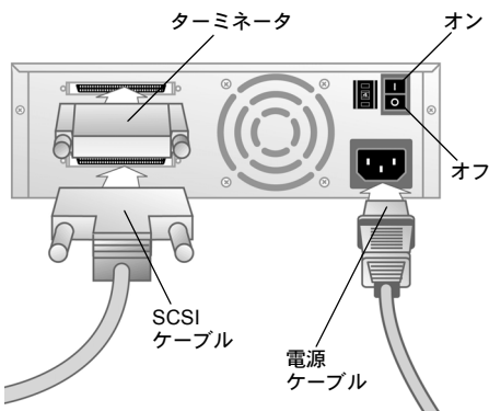
図 3: テープドライブの背面
