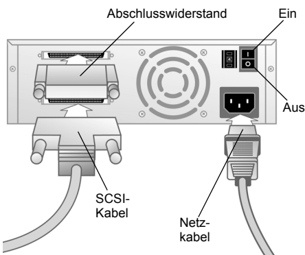
Abbildung 3: Rückseite des Bandlaufwerks
