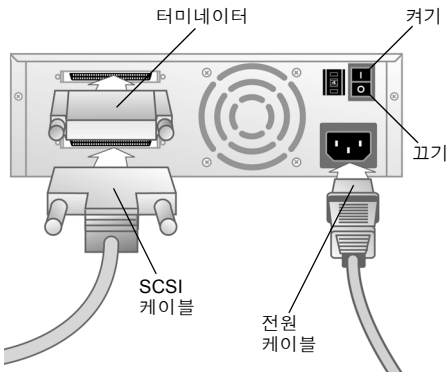
그림 3: 테이프 드라이브 뒷면
