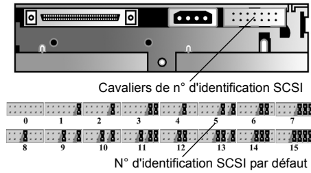
Figure 2 : Installation dans une baie du lecteur
