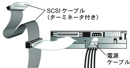
図 5: テープドライブの取り付け
