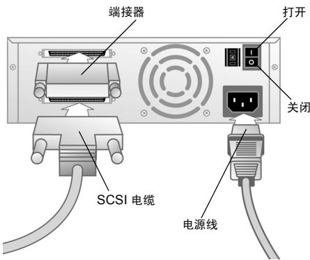
图 3: 磁带驱动器的背面
