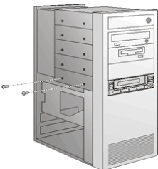
Figura 5: Fije la unidad de cinta
